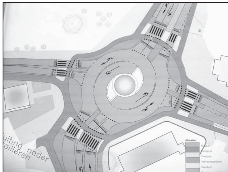
Plan voor de inrichting van rotonde aan het poortlandplein.
